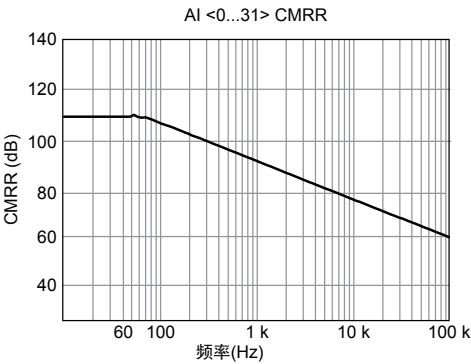
图 2. CMRR, AI+至 AI-
