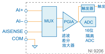
图 1. NI 9206 某模拟输入通道的输入电路
